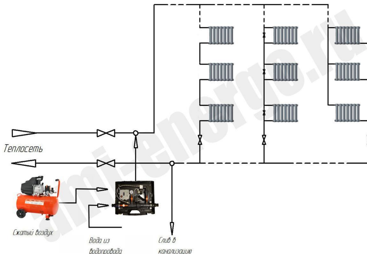
Схема возможного подключения установки «УГП-Микс» при промывке отопления.
